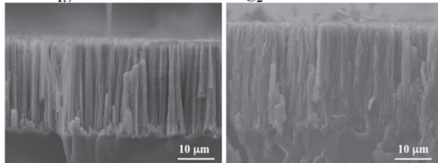
Si基板上に作製したMnSi 1.7 Mg 2 Si ワイヤバンドル
